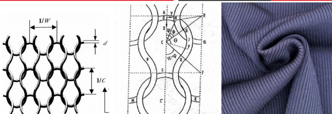
2-rasm. Elastik trikotaj matoning halqa tuzilishi, geometrik modeli va tayyor mato fakturasi
